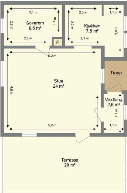
Litjslindvassvegen 161 1. Etasje
