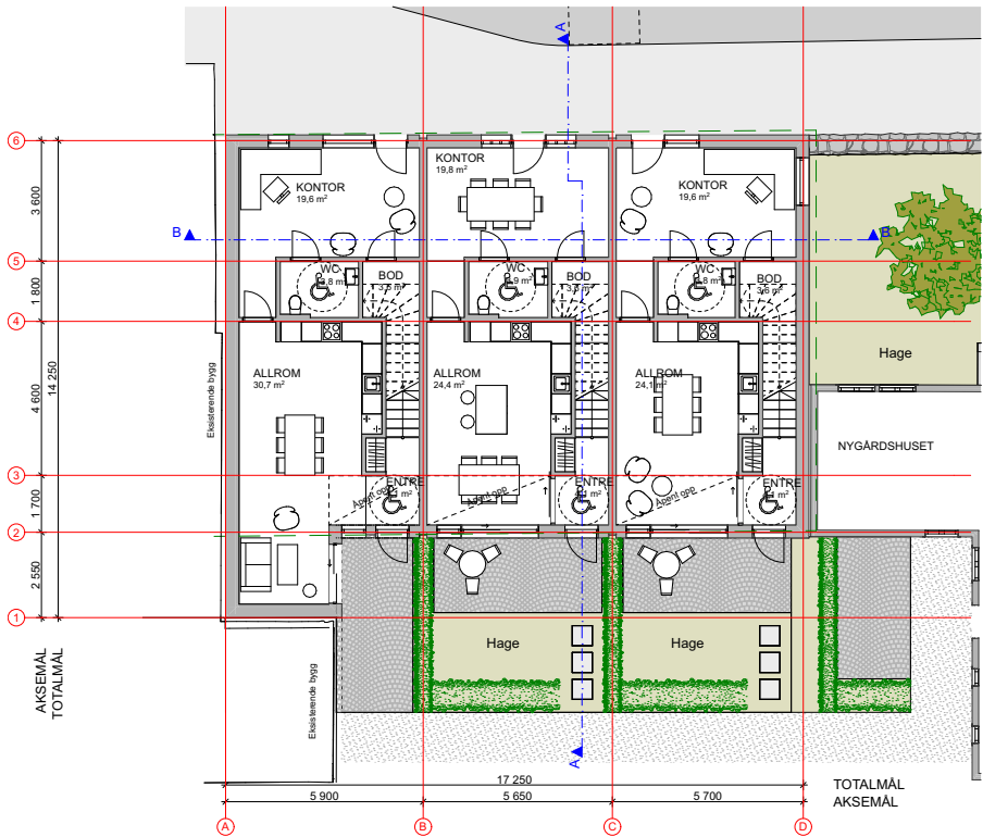
Plan 1. etasje
