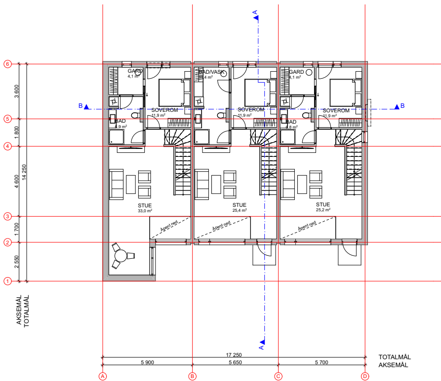
Plan 2. etasje
