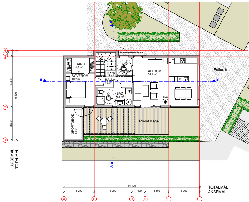
Nygårdshusene AS Gnr 111, bnr 1259 Sandnes sentrum GÅRDHUSET Plan 1.etasje Tegningen er ARC sin eiendom og kan hverken helt eller delvis benyttes til arbeider som ARC ikke medvirker i.
