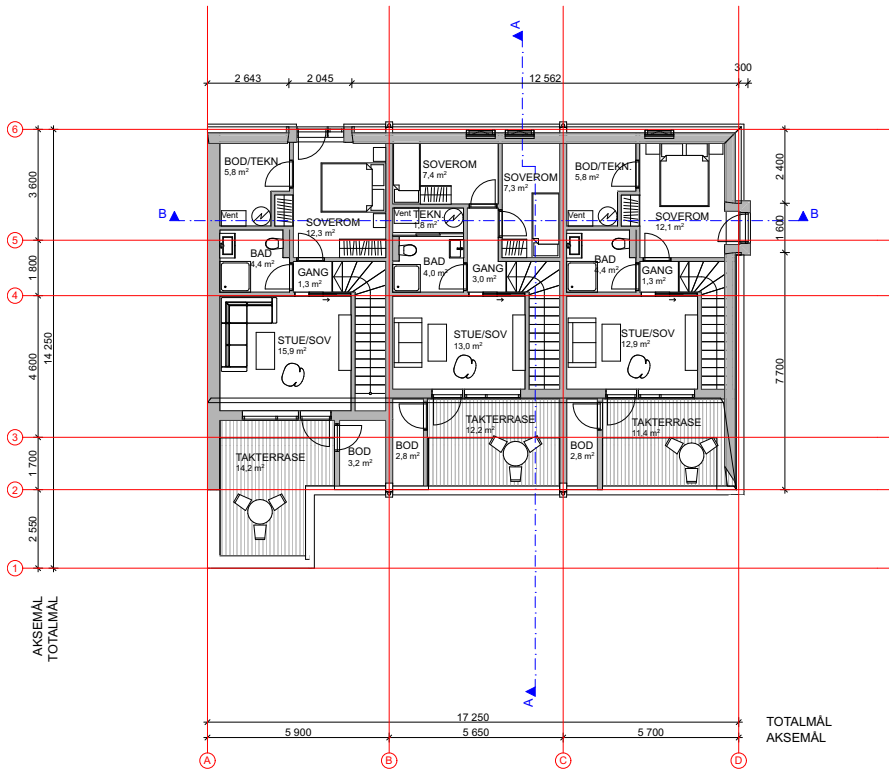
Nygårdshusene AS Gnr 111, bnr 1259 Sandnes sentrum BYHUSENE Plan 3.etasje Tegningen er ARC sin eiendom og kan hverken helt eller delvis benyttes til arbeider som ARC ikke medvirker i.
