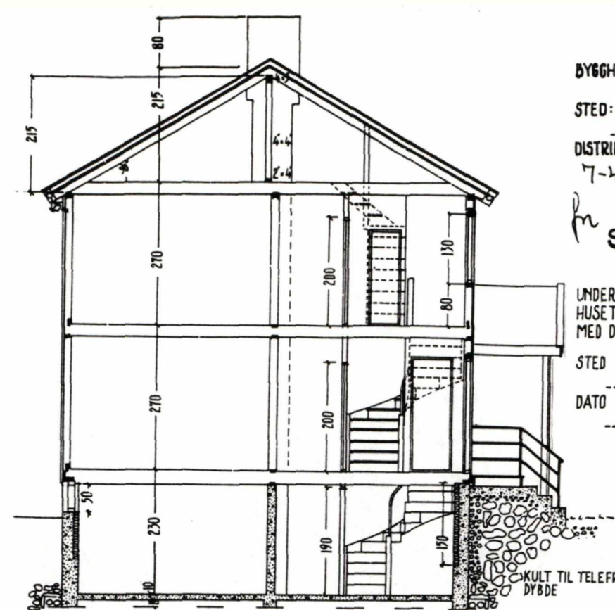
SNITT
