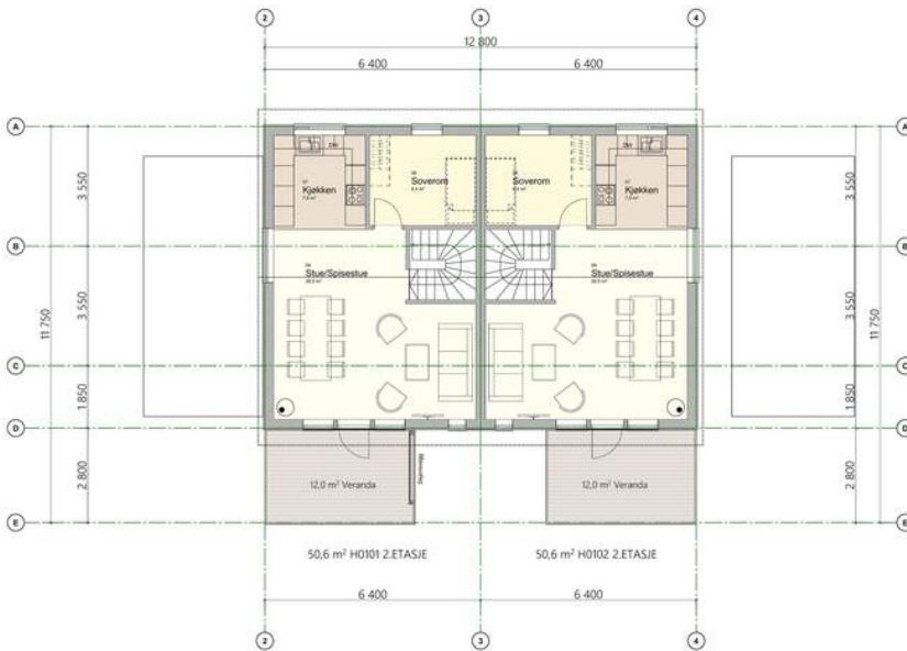
PLAN 2.ETASJE
