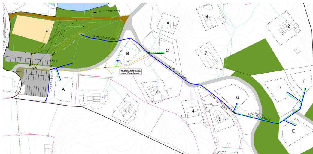
Figur 5. Planlagt ledningssystem
