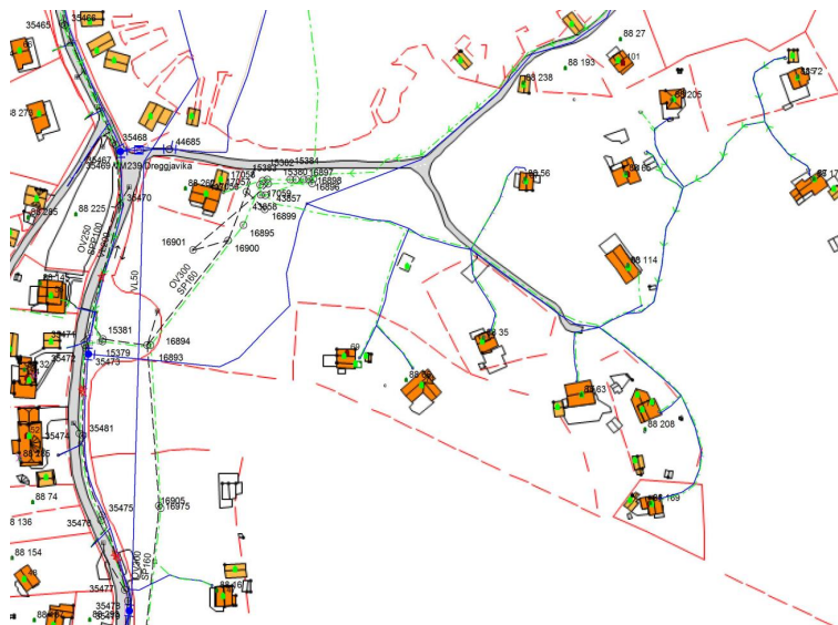
Figur 3. Eksisterende ledningsnett.
