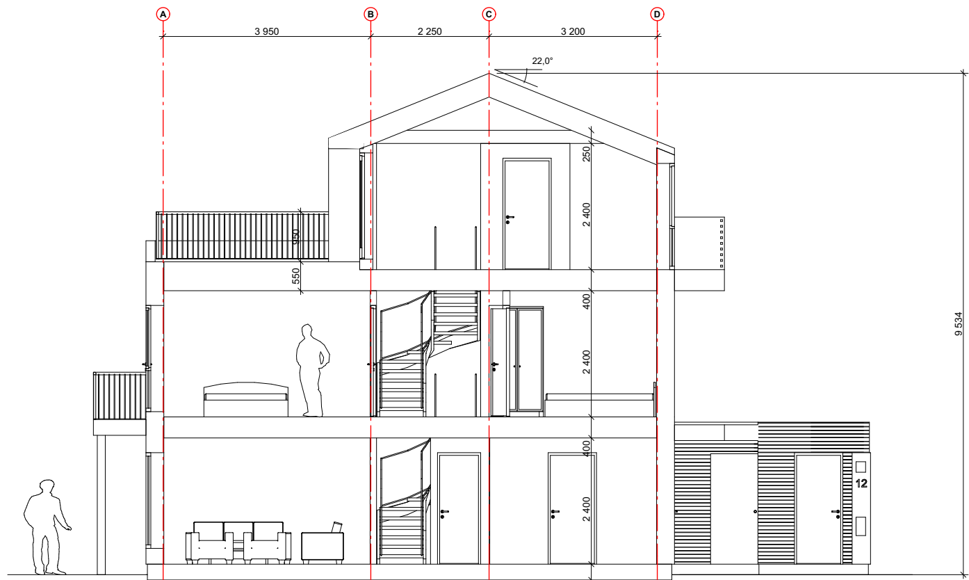
Snitt AA
